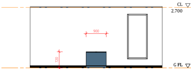
Elevation 6J
