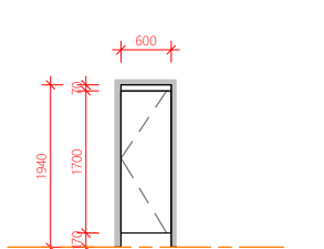
DOOR TYPE K
