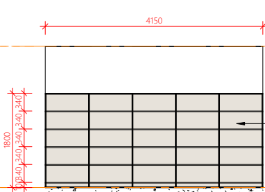
Elevation 6B
