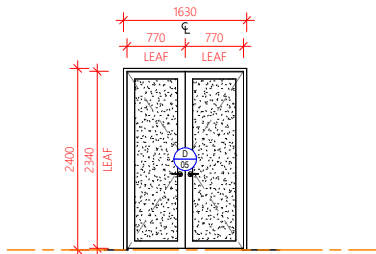
DOOR TYPE B
