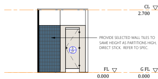
Elevation 4N
