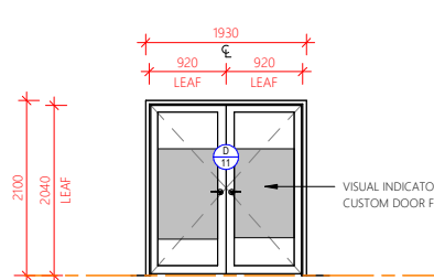
DOOR TYPE C
