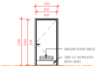
DOOR TYPE F
