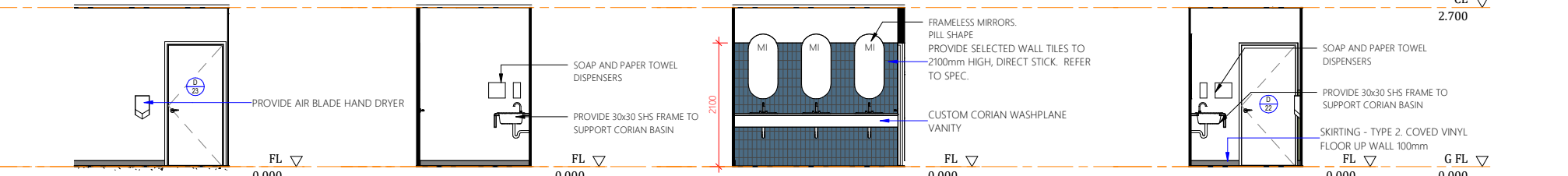
Elevation 4E
