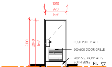
DOOR TYPE G
