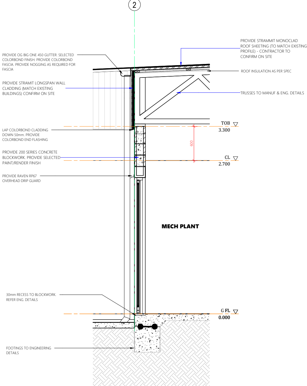
Section Detail D1
