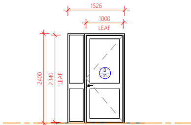
DOOR TYPE A
