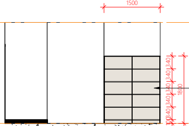
Elevation 6E
