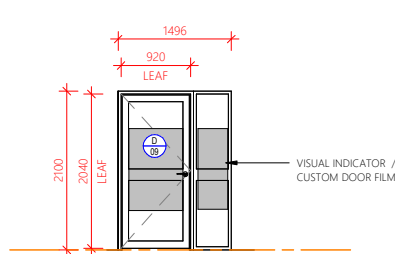
DOOR TYPE D
