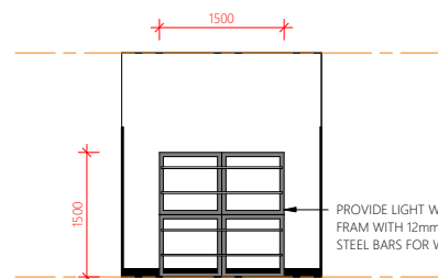
Elevation 6G
